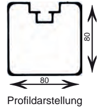
Profildarstellung
